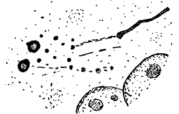
Fig. 3. – Même région. Grossissement 3000:1. Dessin à la chambre claire. Appareil métaterminal en voie de reconstruction après avoir donné naissance à deux rondelles isolées et à des granules de dégénérescence.
