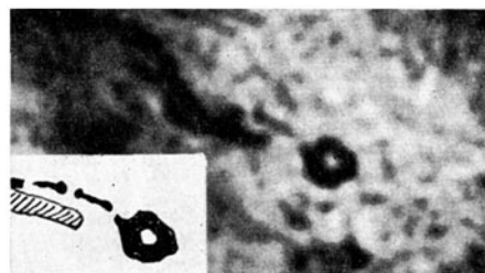
Fig. 2. – Même région, même grossissement. La fibre aboutissant à la rondelle se fragmente.
